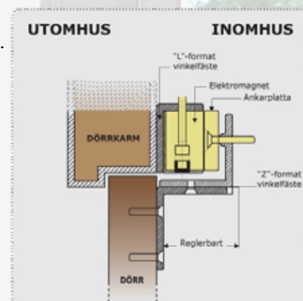
Inåtgående dörr (installerade med "L" och "Z" vinkelfästen).
